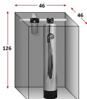
ROZMĚRY SYSTÉMU [cm] - NS3
